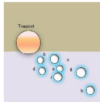
トラピスト-1を周回する7惑
