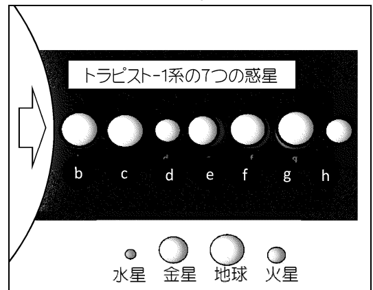
トラピスト-1系の惑星と太陽系惑星の大きさ比較
